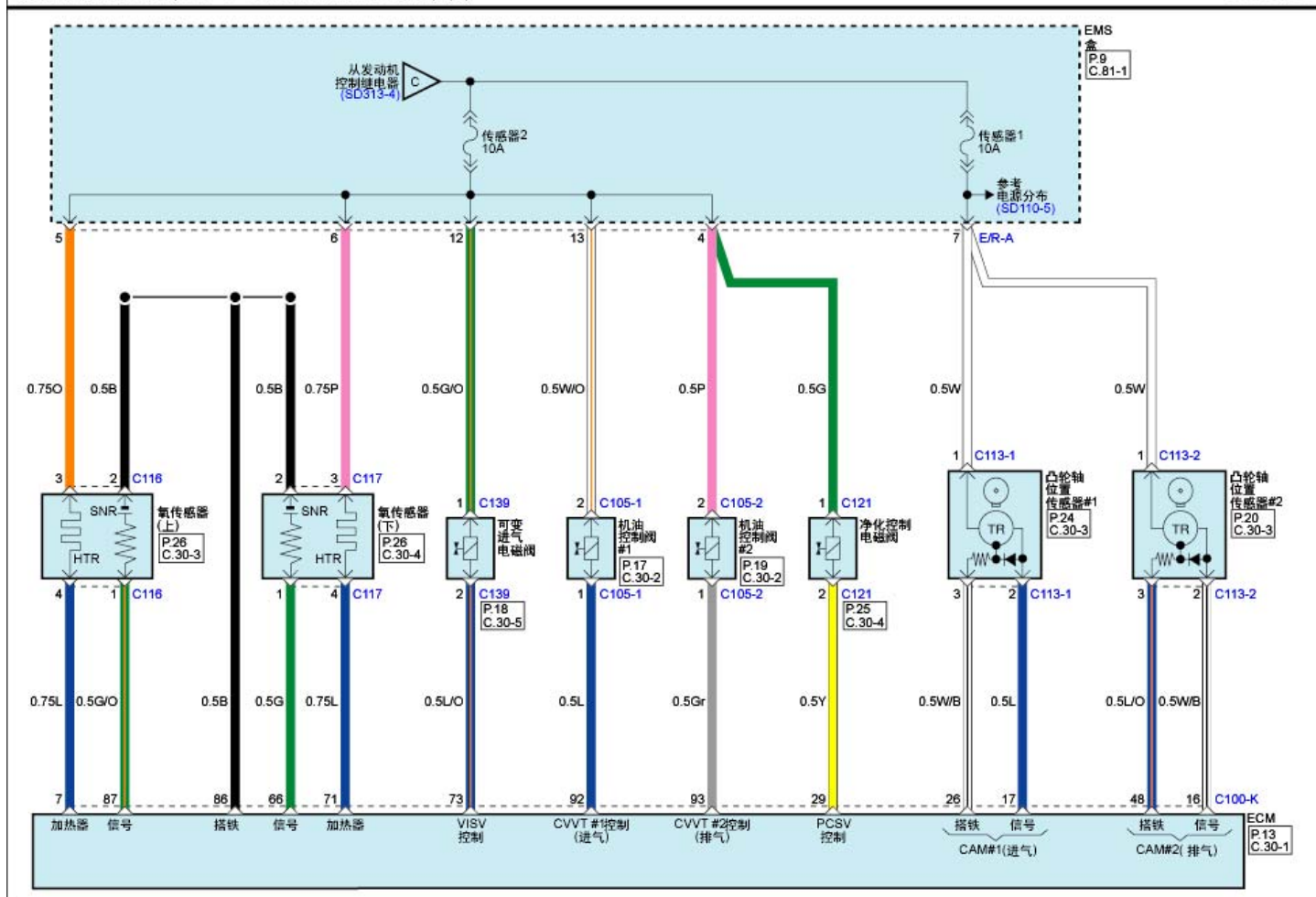
发动机控制系统(G4FG : GAMMA 1.6L MPI) (5)
